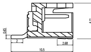
截面 A-A
