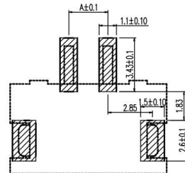
印制线路板
