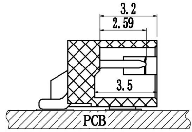
剖面 A-A
