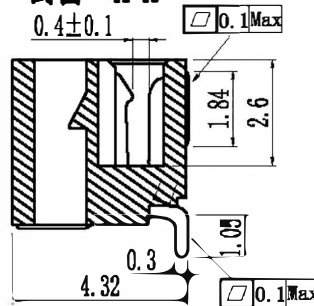
剖面 A-A
