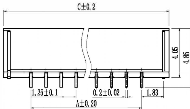
剖面 A-A
